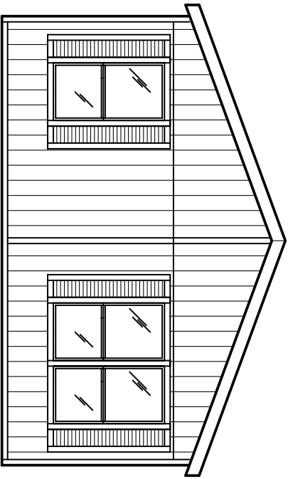
RIGHT ELEVATION
